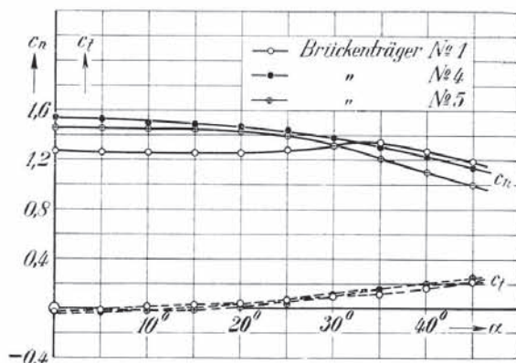
Abb. 126. Wind schräg seitlich.
