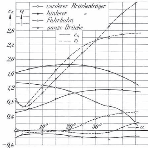
Abb. 130. Wind schräg von oben.
