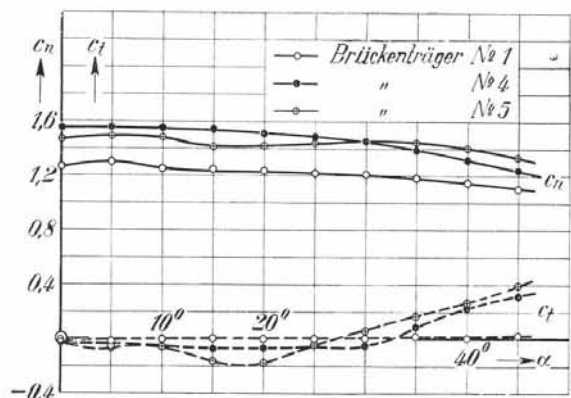
Abb. 125. Wind schräg von oben.
