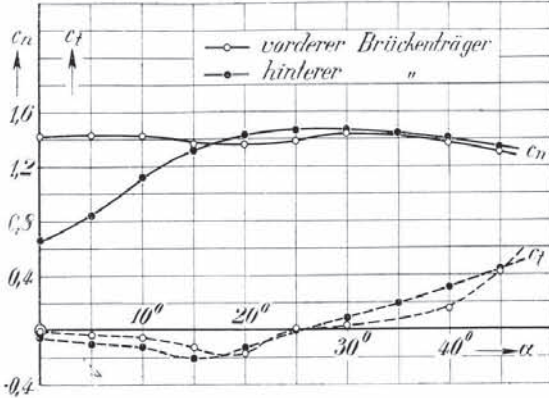
Abb. 128. Wind schräg von oben;
