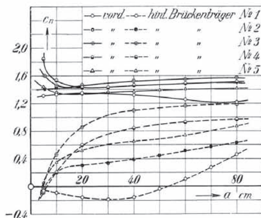
Abb. 127. Wind senkrecht auftreffend.
