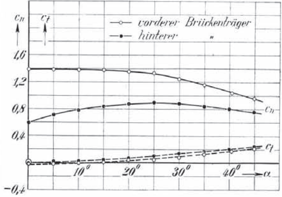
Abb. 129. Wind schräg seitlich.
